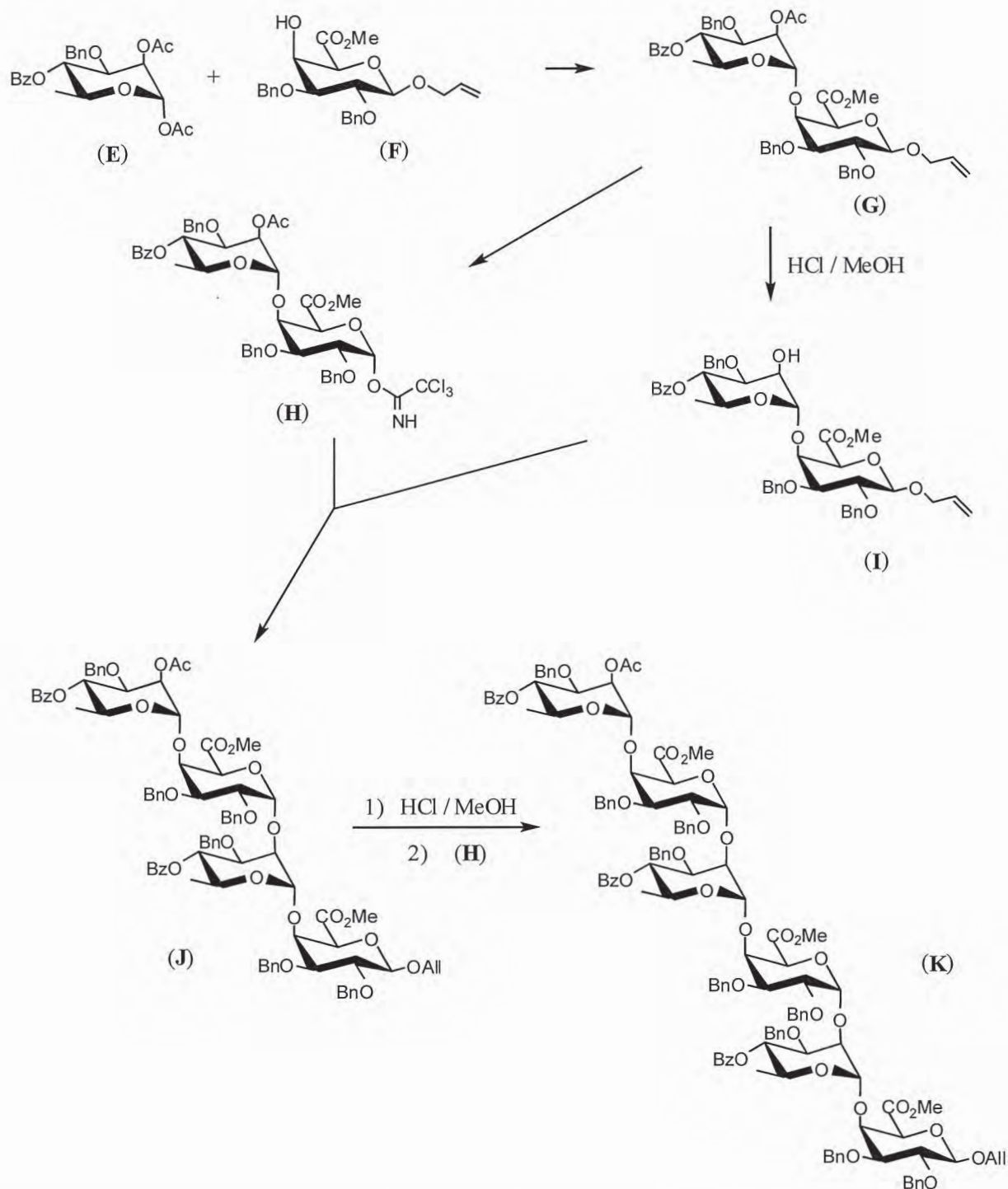
Figure 10. Schéma de synthèse d'un fragment du rhamnogalacturonane (où All = -CH 2 -CH=CH 2 )
